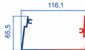
T.2517 1,825 KG/MT Dere Takoza Profili
