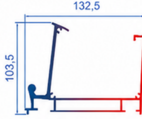
T.2521 3,844 KG/MT Dere Profili
