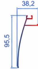
T.2525 0,595 KG/MT Açı Ayar Kapak Profili
