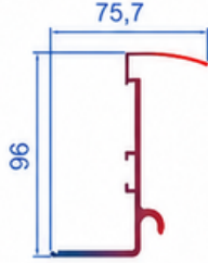
T.2524 1,471 KG/MT Açı Ayar Profili
