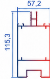
T.2570 2,250 KG/MT Taşıyıcı Ledli Profili
