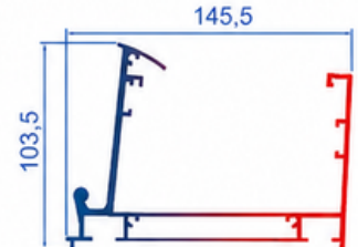
T.2518 4,076 KG/MT Taşıyıcı Dere Profili
