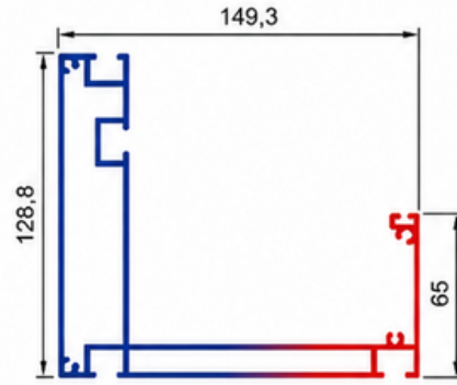
T.2712 - 4,161 KG/MT
