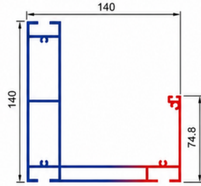
T.2713 - 3,944 KG/MT
