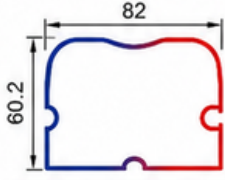
T.2704 - 1,176 KG/MT
