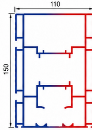
T.2703 - 5,874 KG/MT
