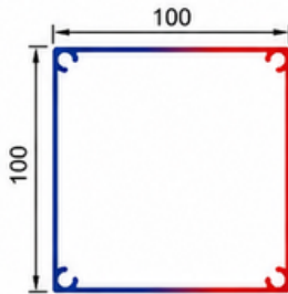
T.2708 - 2,135 KG/MT
