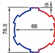
T.2715 - 1,057 KG/MT
