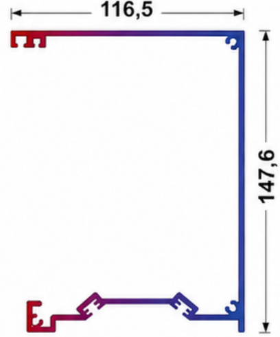
T.2401 - 3,182 KG/MT
