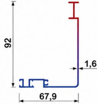
T.2478 - 0,959 KG/MT
