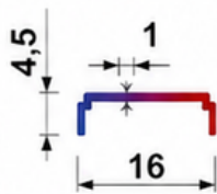
T.9105 - 0,060 KG/MT
