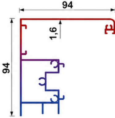
T.2477 - 1,856 KG/MT
