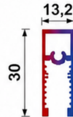
T.2410 - 0,400 KG/MT
